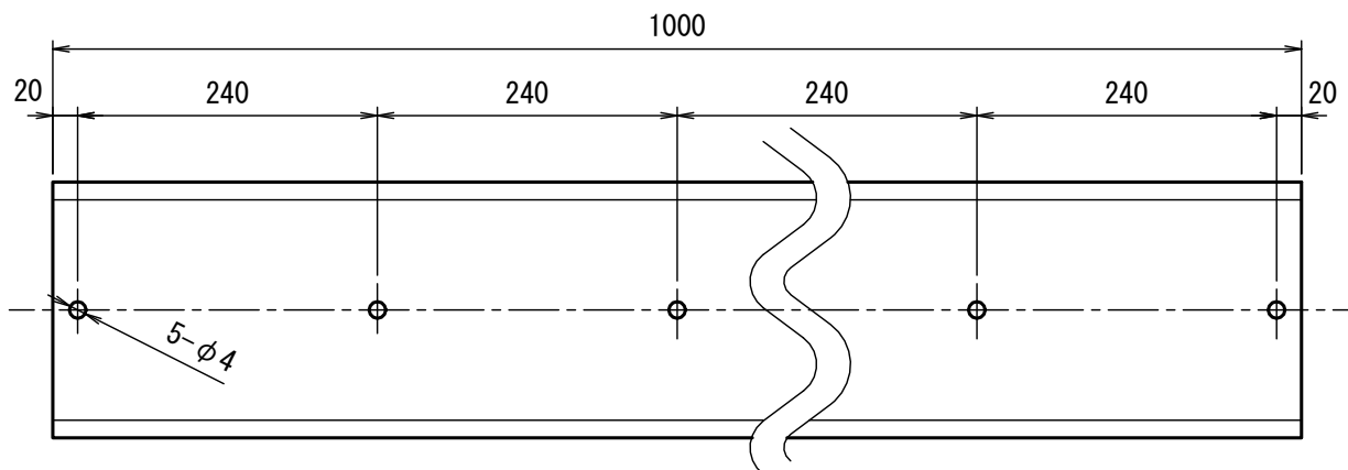
釘穴加工図
